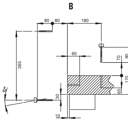
Fresa supplementare / Unità a forare Fraise supplémentaire / Unitè de perçage Additional milling unit / Drilling unit Cabezal fresador suplementario / Unidad a taladrar
