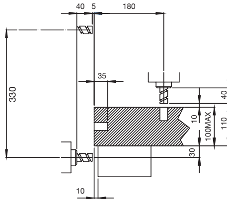
Fresa supplementare Fraise supplémentaire Additional milling unit Grupo fresa suplementario
